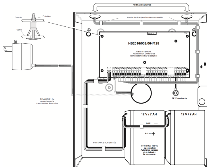
Figure 2-1 Acheminement du câblage (Amérique du Nord uniquement)
