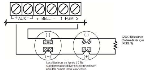
Figure 2-15 Câblage d'un détecteur de fumée à 2 fils
