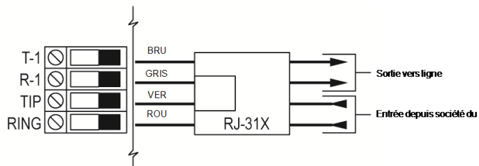
Figure 2-13 Câblage de ligne téléphonique
