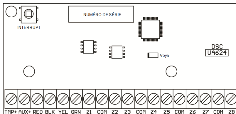
Figure 2-3 Extenseur de zone HSM2108
