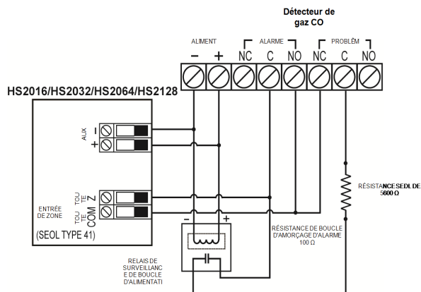
Figure 2-16 Câblage de détecteur de gaz CO
