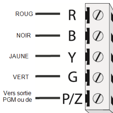
Figure 2-7 Bornes P/Z de clavier
