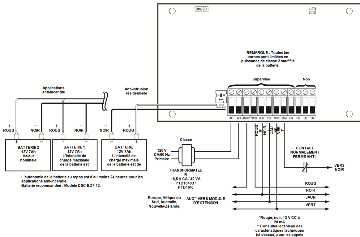
Figure 2-6 Câblage d'une alimentation électrique
