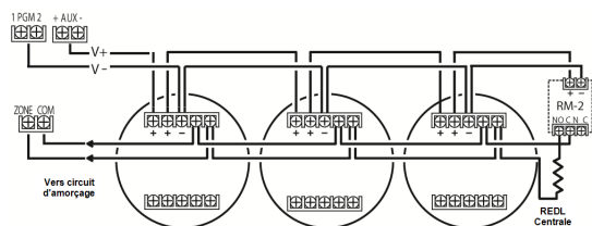
Figure 2-14 Câblage de détecteur de fumée
