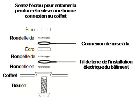
Figure 2-17 Mise à la terre
