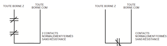
Figure 2-8 Normalement fermé
