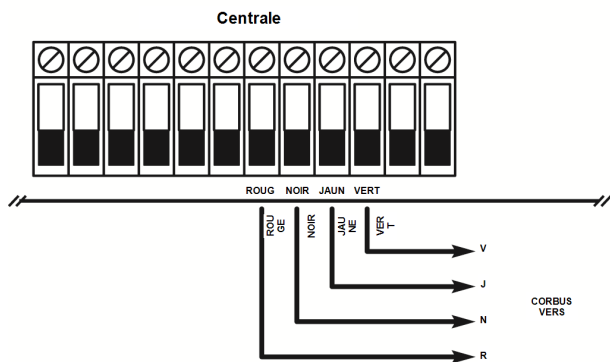
Figure 2-5 Schéma de câblage du système HSM2HOSTx
