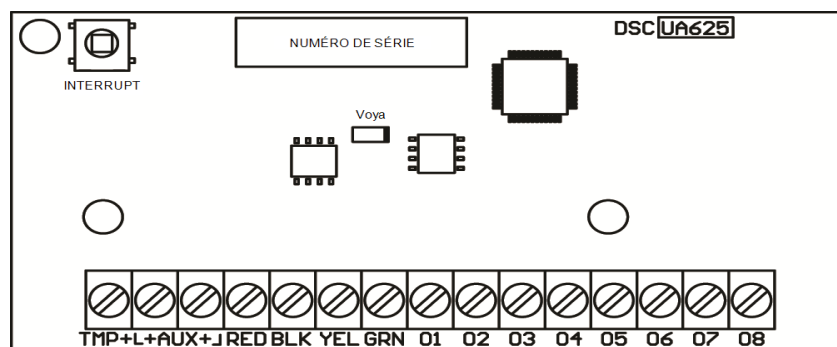
Figure 2-4 Extenseur de sorties HSM2208
