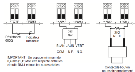
Figure 2-11 Sortie de voyant à résistance de limitation de courant et sortie à étage de relais facultative.
